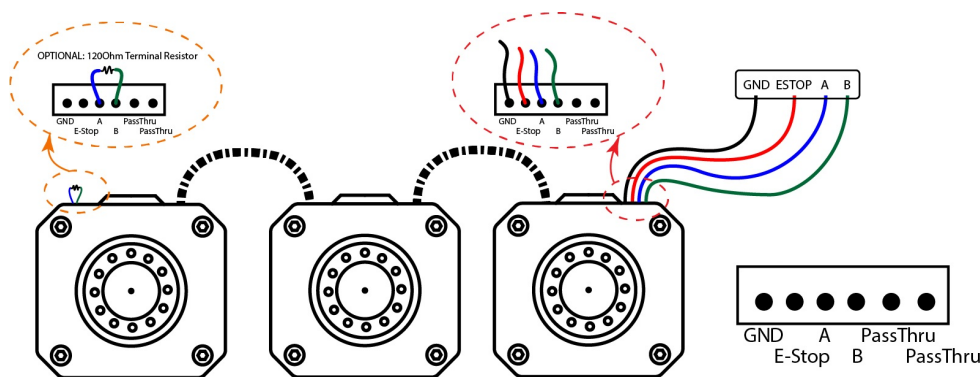
图 9: BEAR 的菊花链串接
