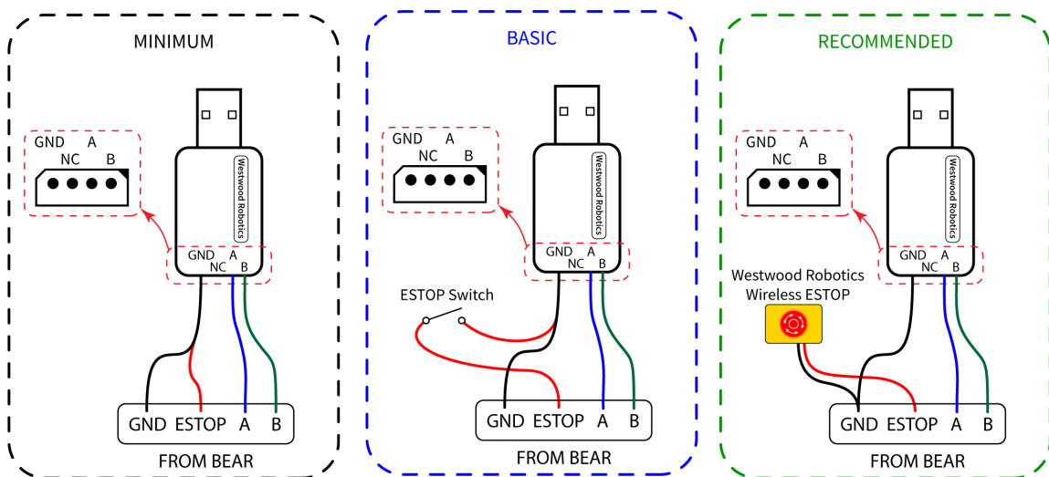
图 11: BEAR 与 USB2BEAR 的连接方法
