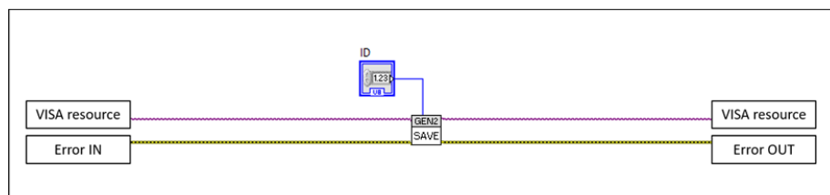
图 18: 保存配置寄存器
