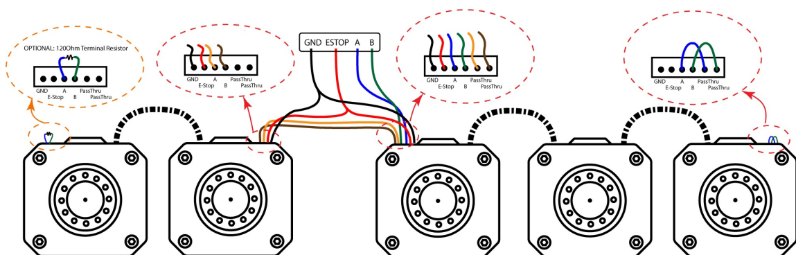
图 10: BEAR 的分叉链接
