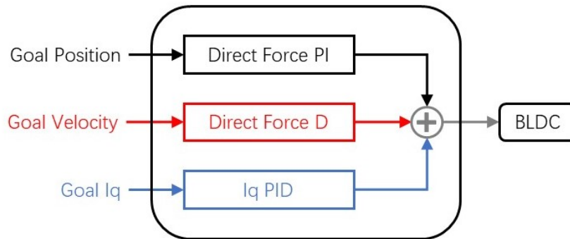
图 12: Direct Force Mode 示意图.
