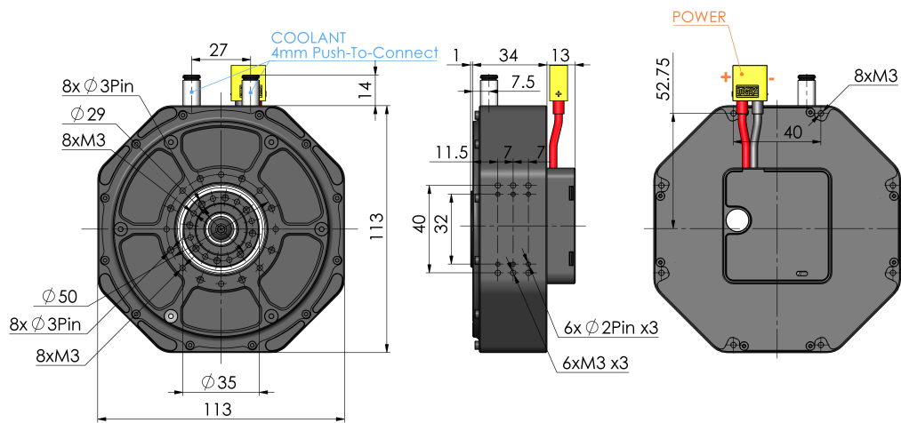
图 3: Panda BEAR V2 Specs
