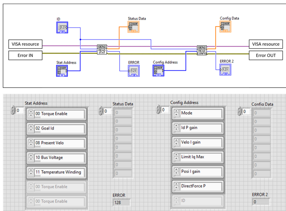
图 16: 数据读取
