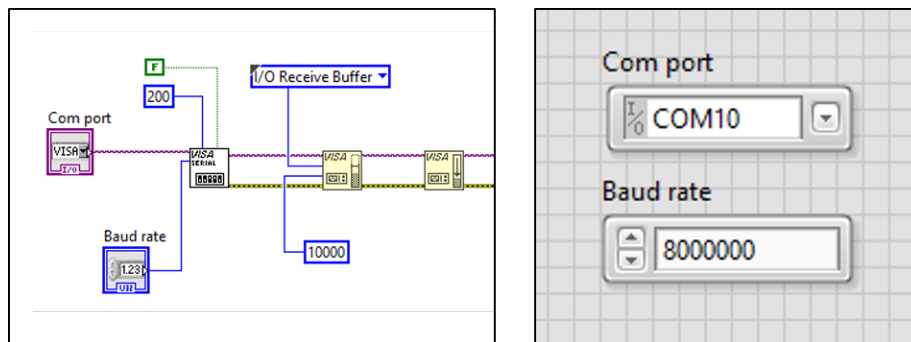
图 15: 打开一个与 BEAR 通信的 VISA 端口。
