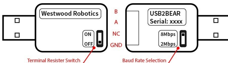
图 8: USB2BEAR 接口引脚标注以及开关
